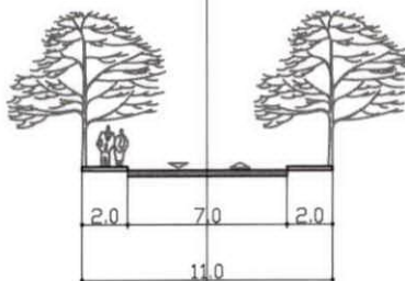
presjek 4-4
